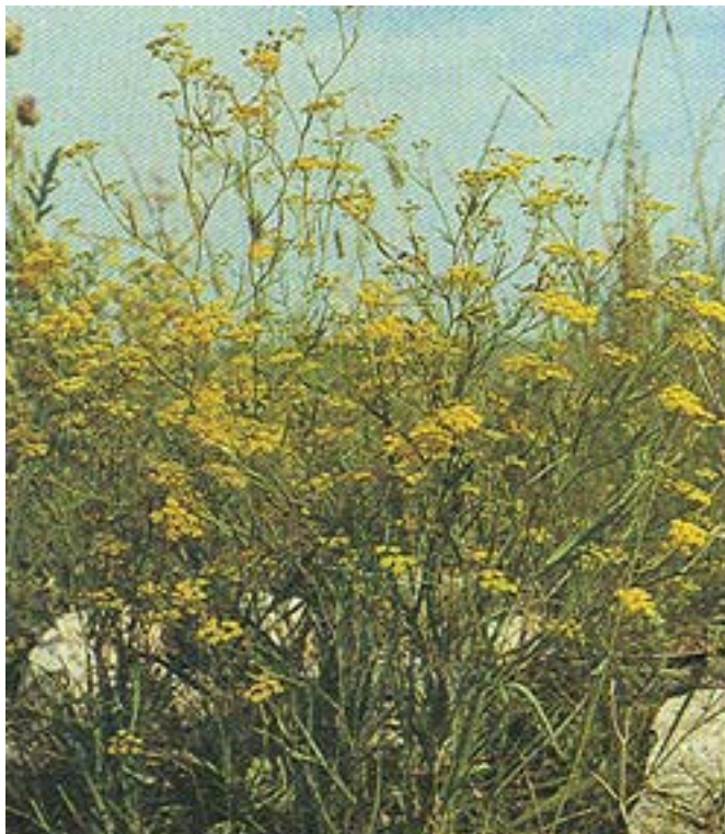
Bupleurum scorzoneraefolium
